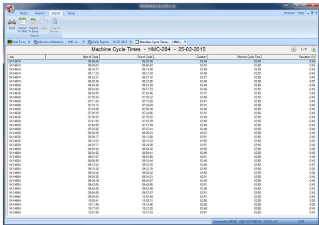
Maschinennutzung (mit wählbarer Sortierung)
