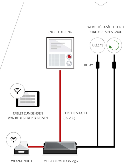
BEISPIEL FÜR EIN DRAHTLOSES NETZWERK MIT HARDWAREVERBINDUNG UND MDC-BOX/MOXA IOLOGIK
