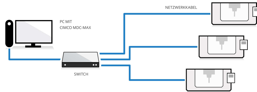
BEISPIEL FÜR EIN KABELNETZWERK MIT DIREKTER VERBINDUNG DER MASCHINEN
